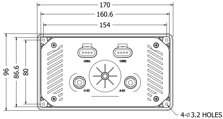
후면도(마운팅 홀 위치)
